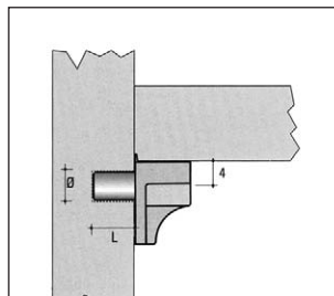
ME13 Csapos polctartó anyag: fém-műanyag
