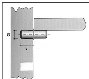
37117 Csapos polctartó felület: horganyzott méret: \varnothing 5 \times 16 mm 00013600002
