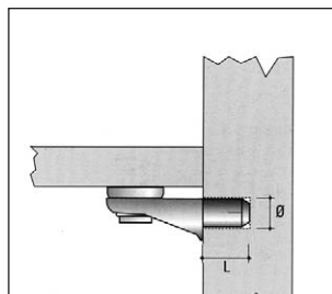
MV01 Csapos üvegpalc tartó anyag: fém-műanyag
