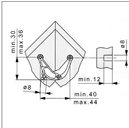
Párkány összehúzó anyag: cink öntvény rendelés: db 00003309000
