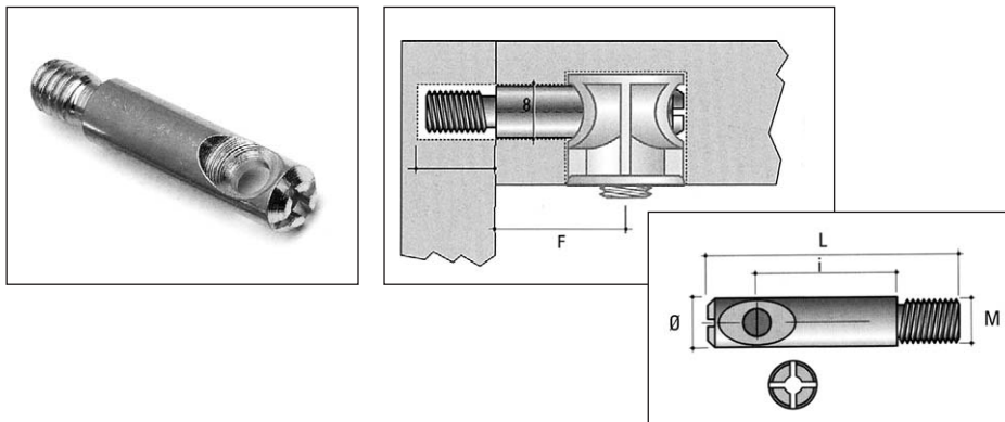
TF03 Összekötő szár, M6 felület: horganyzott 00003310090
