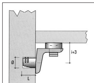
MV03 Körmös üvegpalc tartó anyag: fém-műanyag
