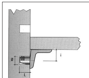
ME05 Körmös polctartó
