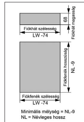
A fiókhát és fenék méretei v = 16 mm!
