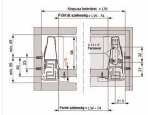
Szerelési méretek 86 mm magas fiókoldal alkalmazása esetén
