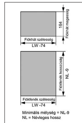
A fiókhát és fenék méretei v = 16 mm!
